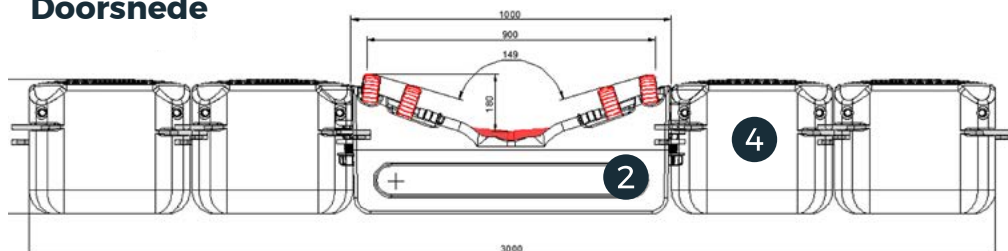
Doorsnede
