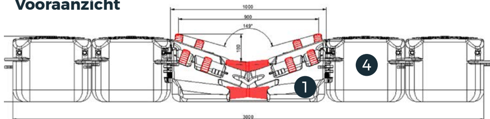
Vooraanzicht
