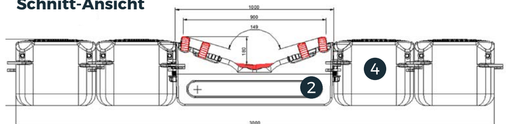
Schnitt-Ansicht
